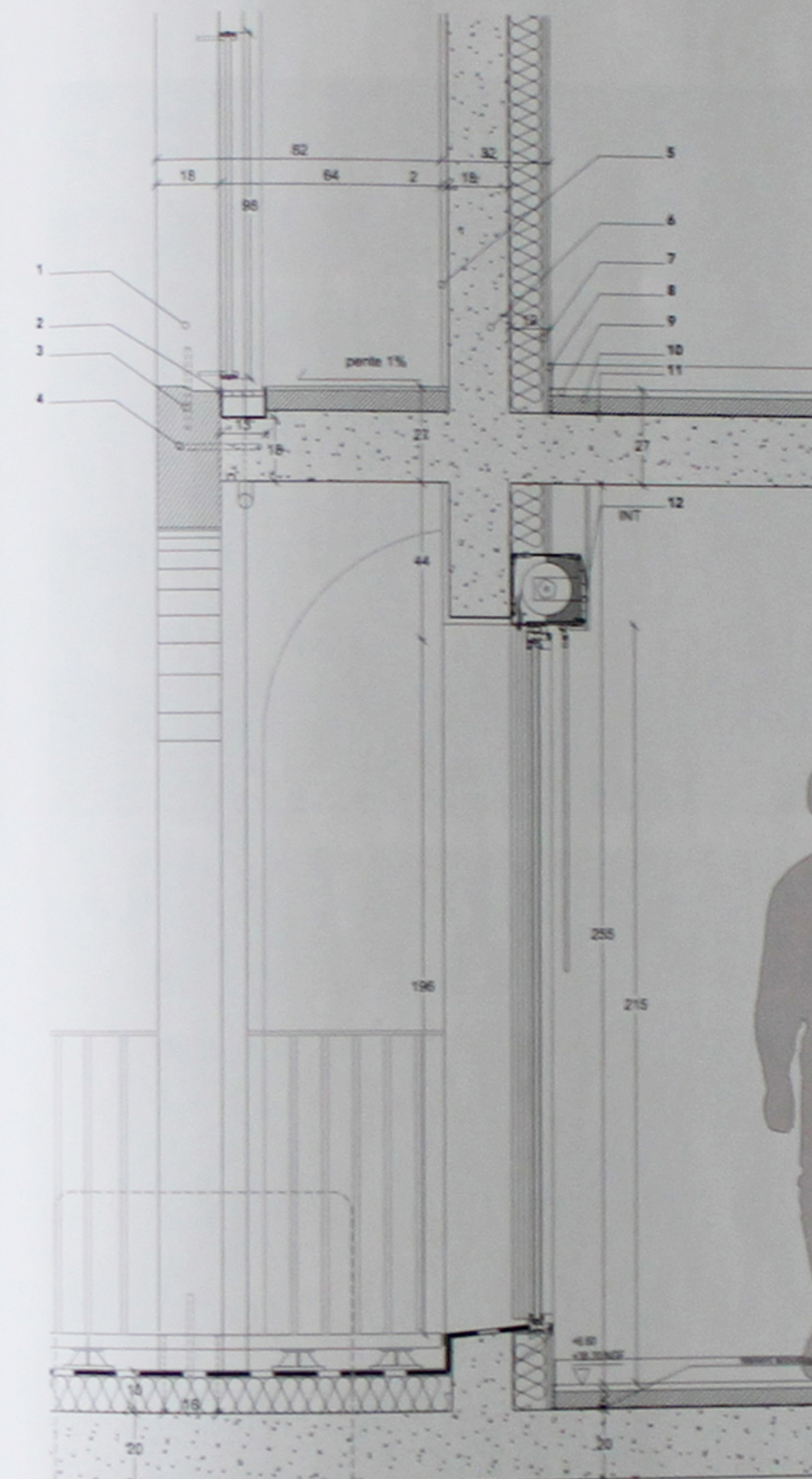
DÉTAIL FAÇADE
